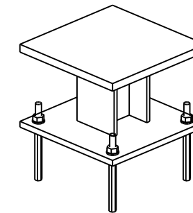
Widok 3D
