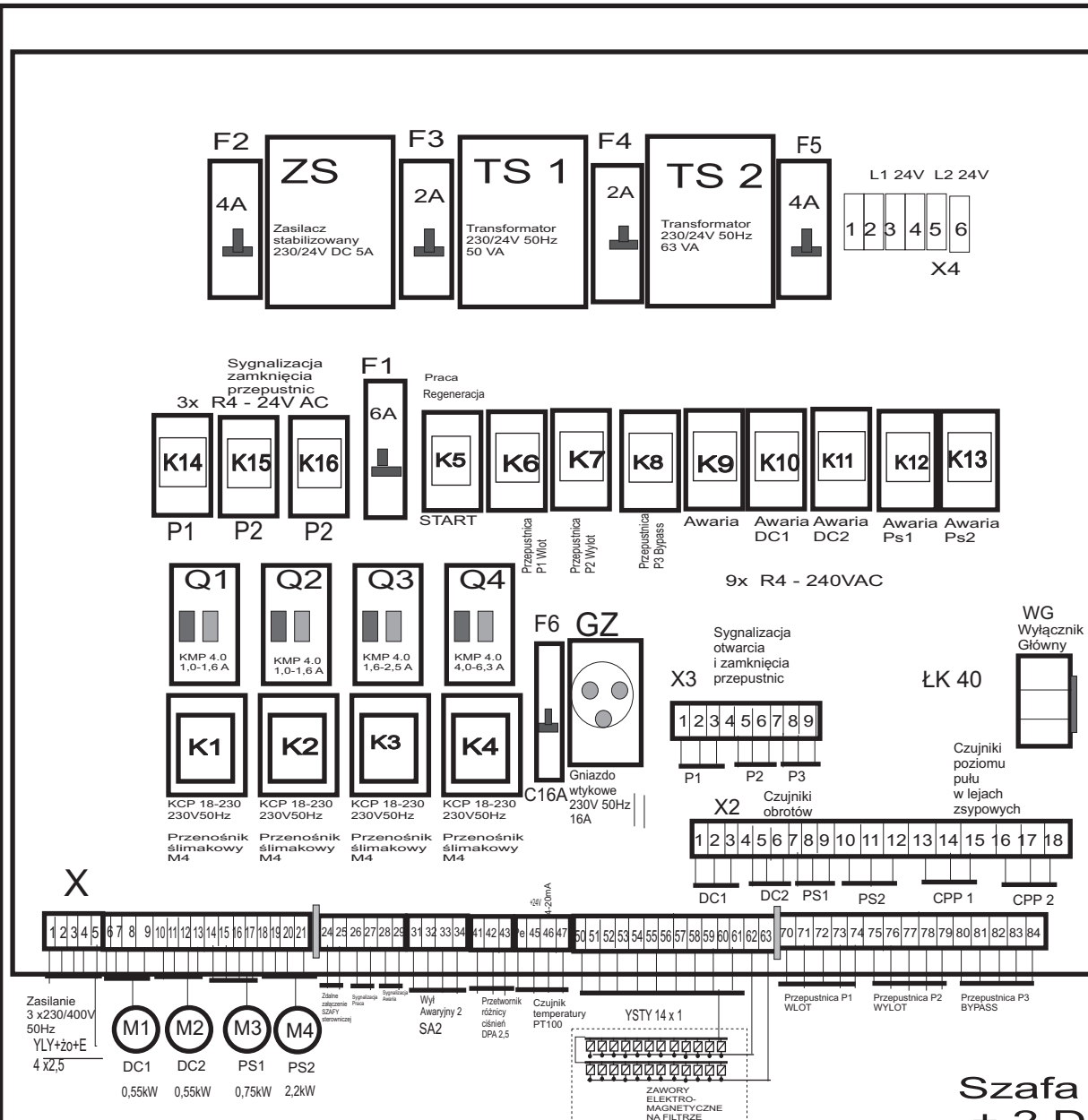
Rys 2 Schemat montażowy
